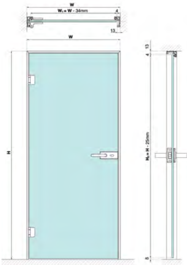
L-Type Door Frame
